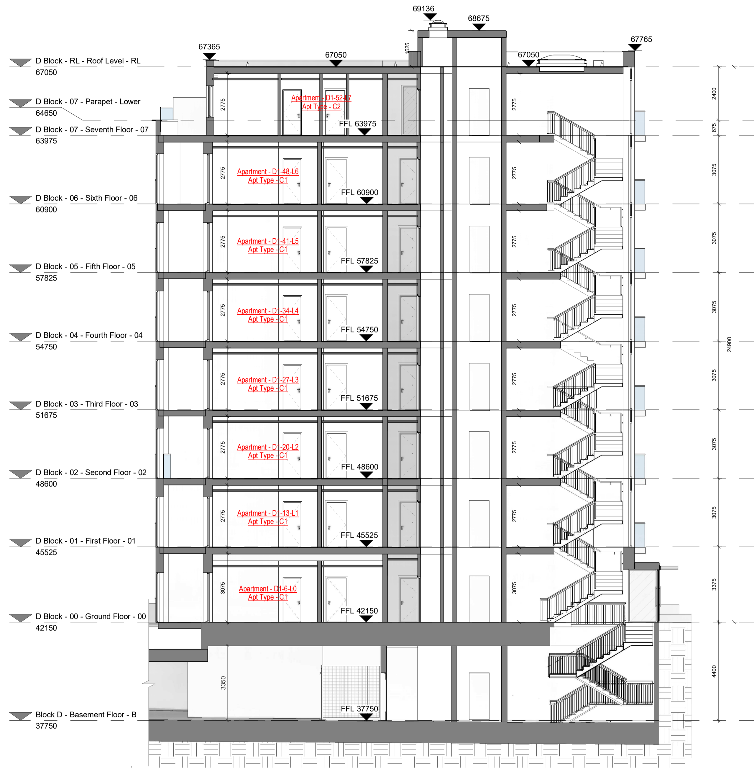
1 GA - Section BB 1 : 100
