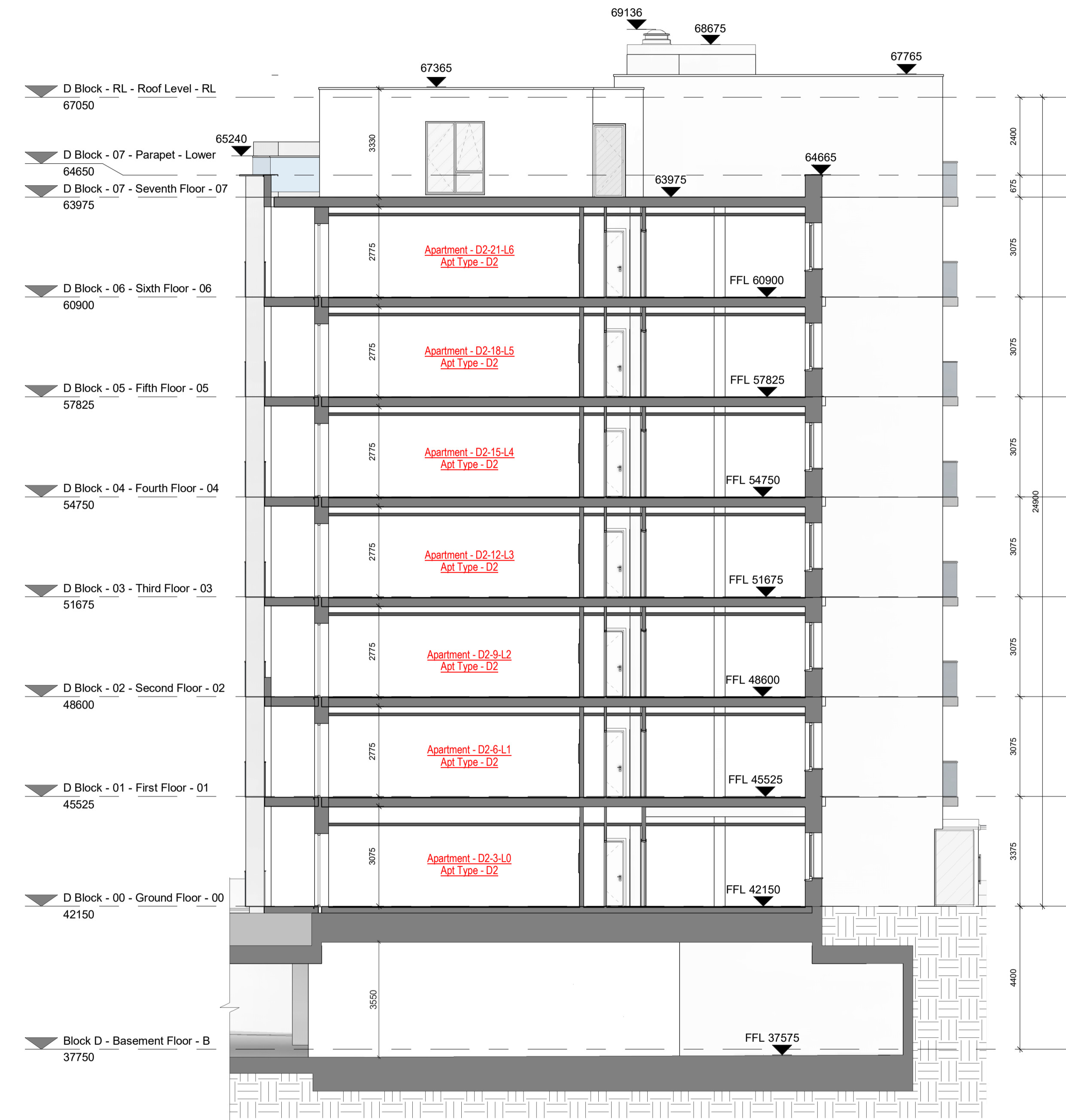
2 GA - Section CC 1 : 100
